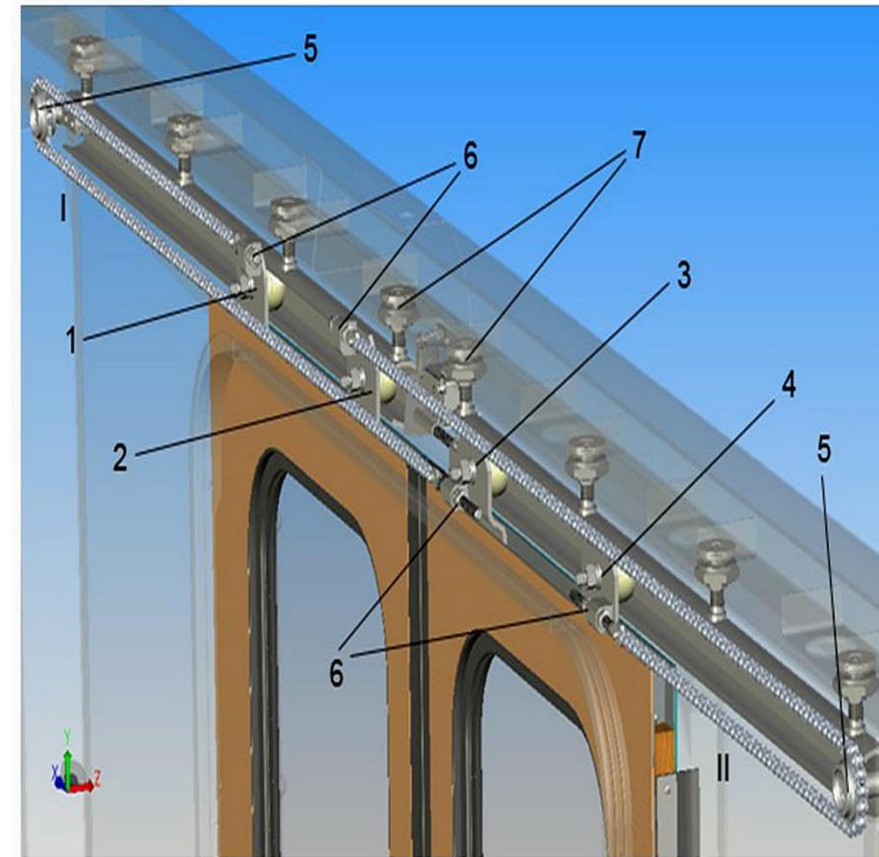
Рис. 3.14. Цепной механизм
