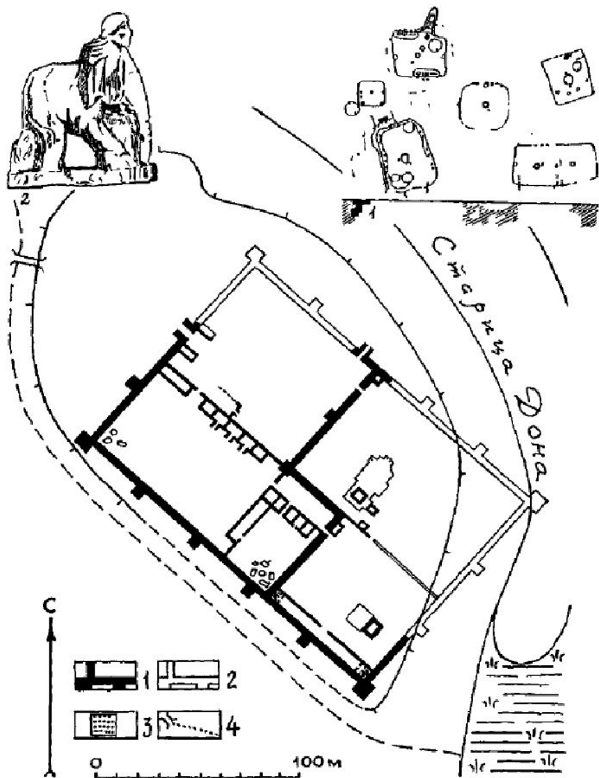
Рис 26 План Саркела. На врезке 1 — план "таборного" или куренного построения (по кругу) двора или "лагеря", обнаруженного в центральной части крепости. На врезке 2 — шахматная фигурка слона, очевидно, потерянного хозяином жилища, входившего в "курень". Условные обозначения: 1 — расчищенные следы кирпичных кладок стен крепости, 2 — не раскопанные или уничтоженные старицей участки стен, 3 — замощенные кирпичом площадки, 4 — предполагаемые дорога и мост через проточный ров.
