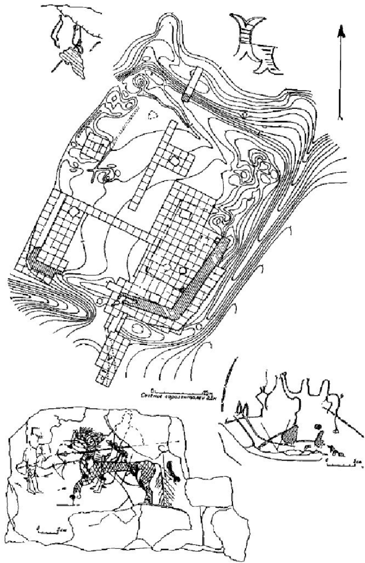
Рис. 21. План Маянкой крепости и раскопов на ней. Вокруг плана размещены рисунки на блоках крепостной стены
