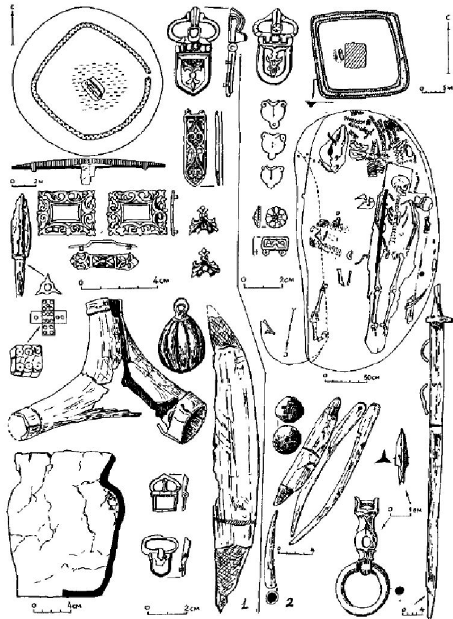
Рис. 33. Два близких по времени кургана: курган так называемой "Веселовской группы", расположенной в регионе Нижнего Дона—Маньча (1); курган из курганной группы "Кривая Лука", расположенной в районе Нижней Волги (2)
