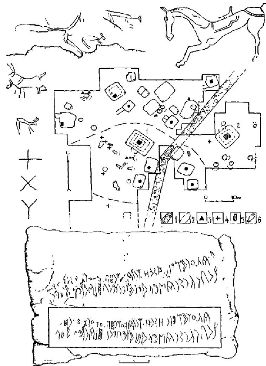
Рис. 22. План части раскопа на поселении, на котором выявлено два святыхища с типологически различными катакомбами вокруг каждого. Как на предыдущих рисунках, вокруг плана размещены различные изображения, открытые на стенах крепости и на отдельных блоках. Особенный интерес представляет двухстрочная руническая надпись (пока не прочтенная)
