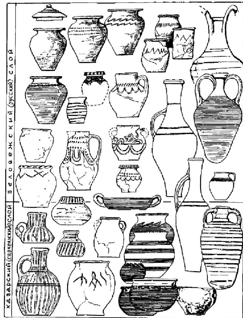
Рис 28. Керамика, характеризующая хазарский и русский периоды жизни Саркела — Белой Вежи.
