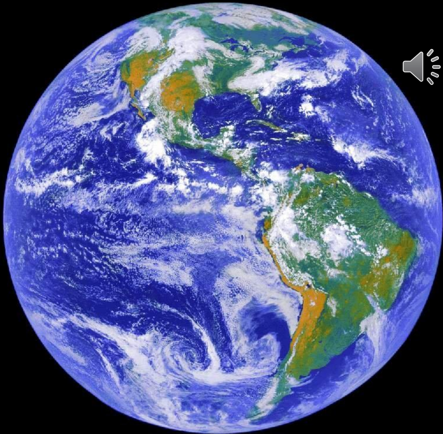
earth
