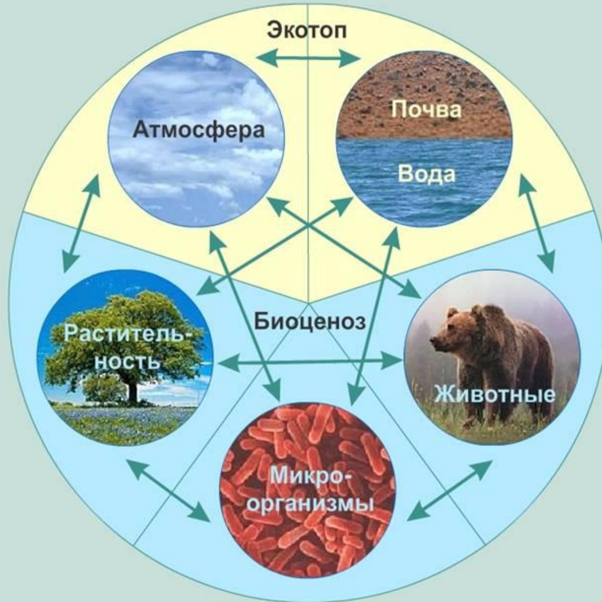
Схема биогеоценоза.
