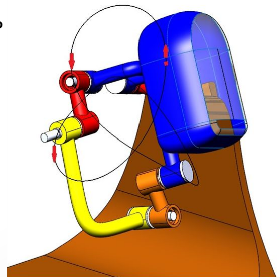
Ведущий стержень
