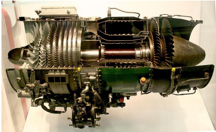
Газотурбінний
