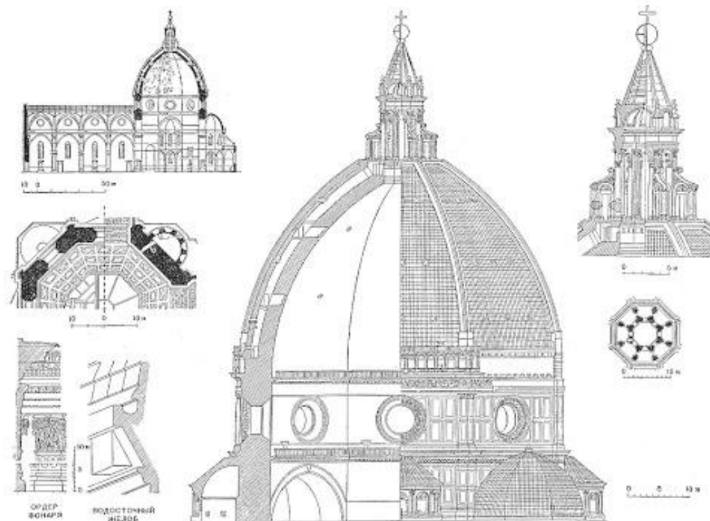
Флоренция. Собор Санта Мариа дель Фьоре, 1296—1470 гг. Продольный разрез; купол и его детали
