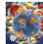
Вирус иммунодефицита
