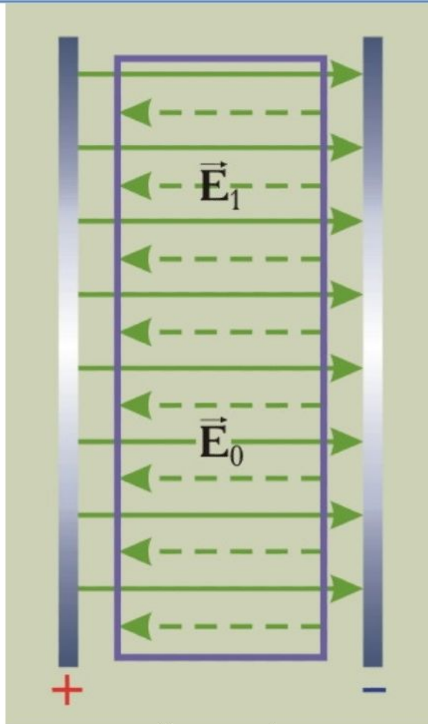
Сложение полей.
