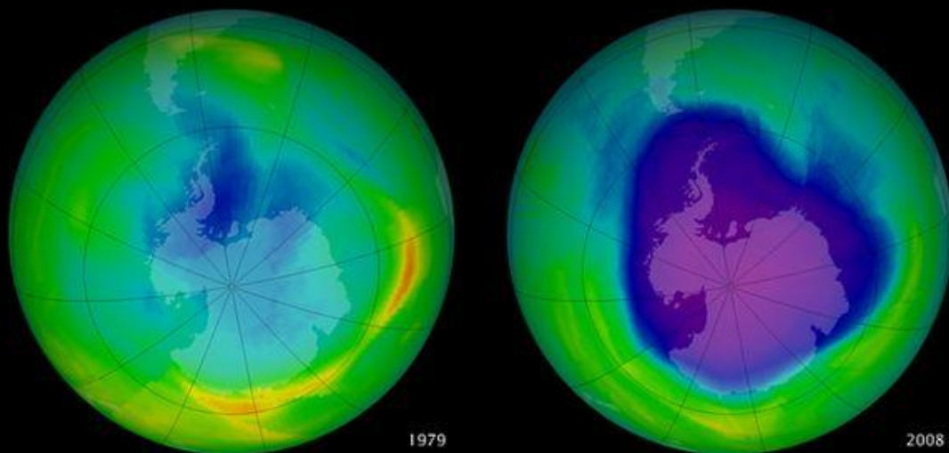
Озоновая дыра над Антарктидой в 1979 и 2008 годах (данные НАСА)
