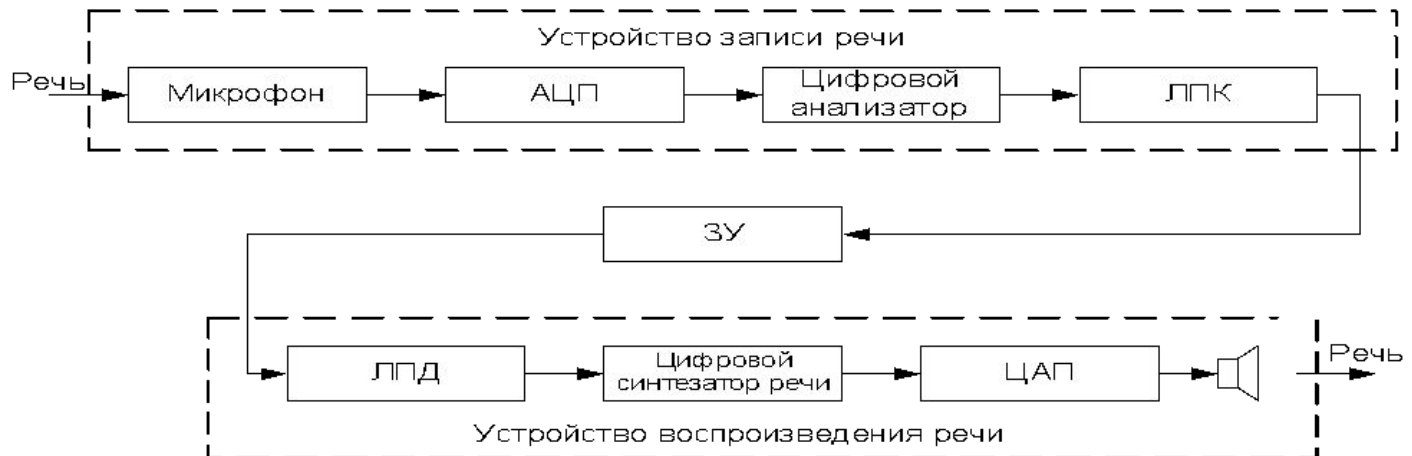
Схема синтеза речи по методу линейного предиктивного кодирования
