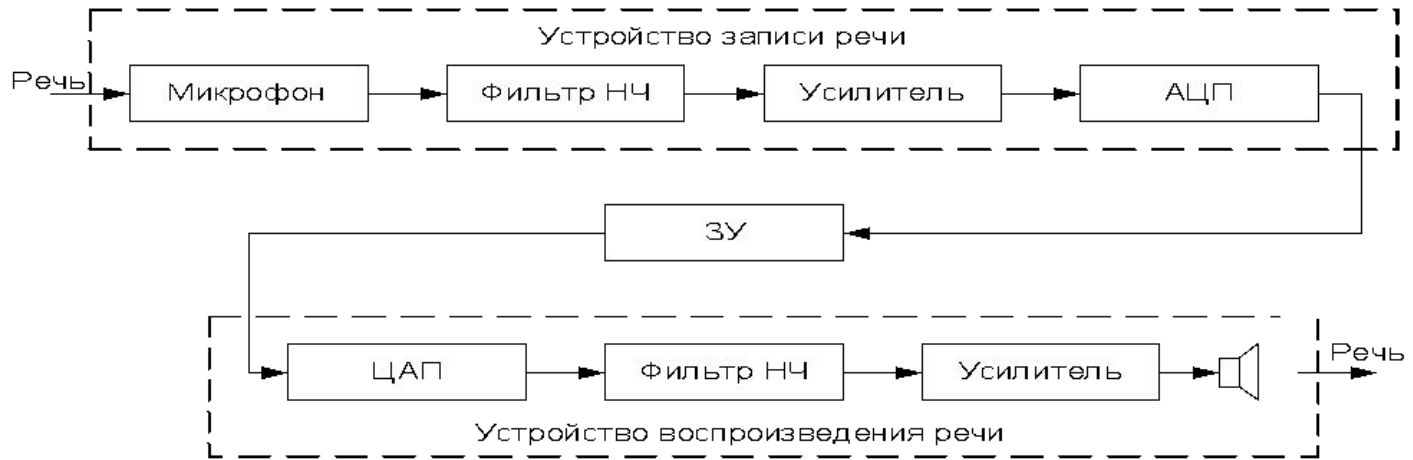
Схема синтезатора речи с непосредственным кодированием – восстановлением сигнала
