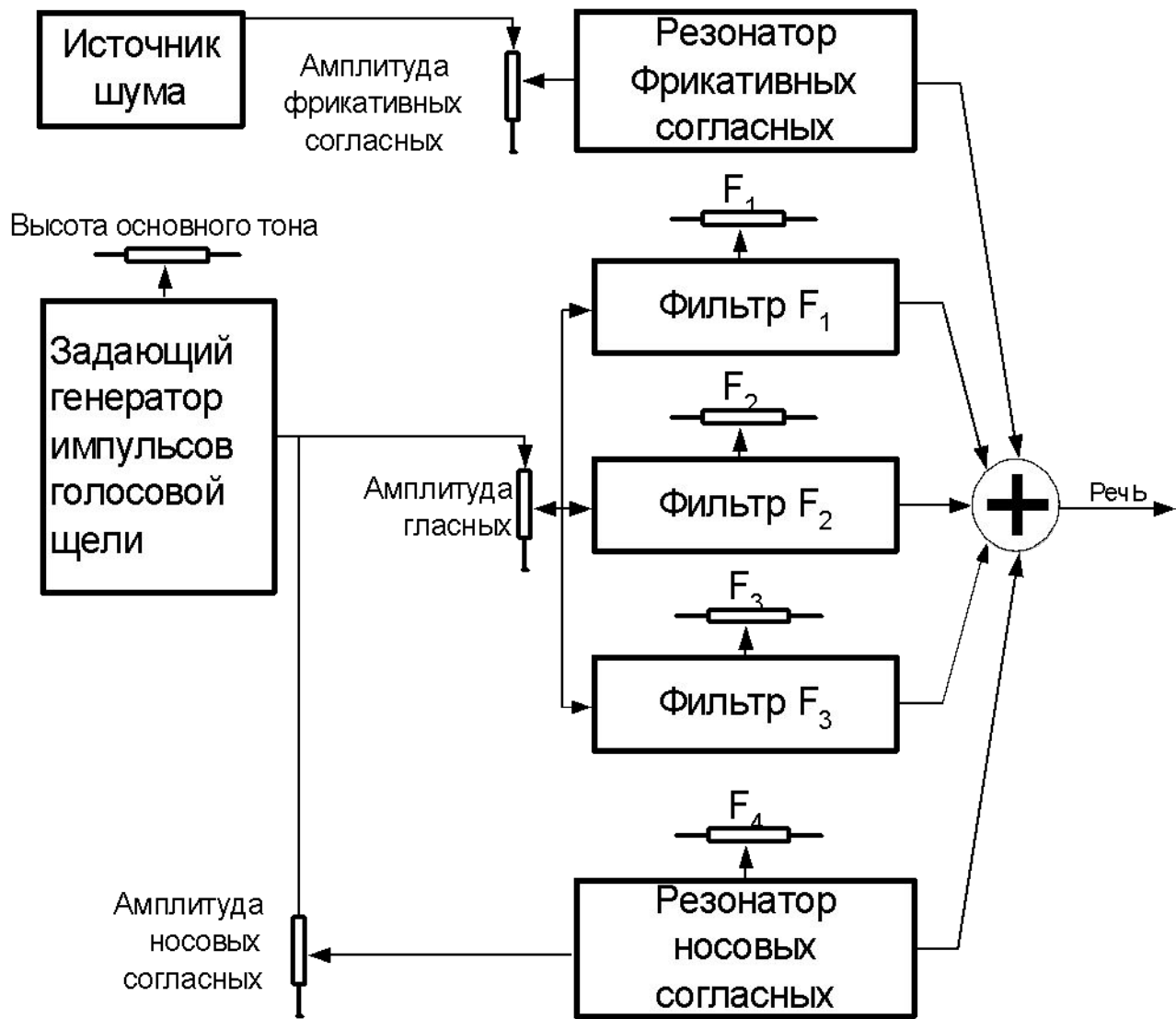
Схема формантного синтезатора речи
