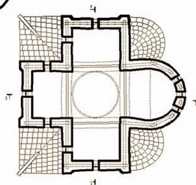
ПЛАН 2 ЯРУСА
