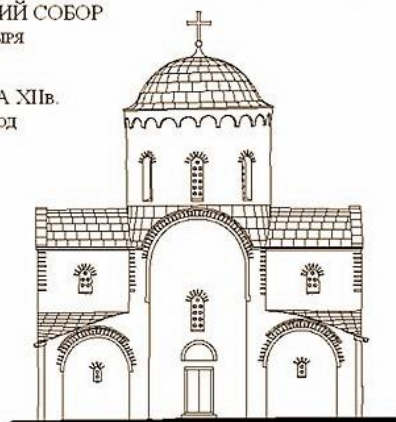
ЗАПАДНЫЙ ФАСАД
