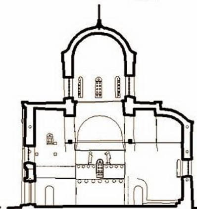
РАЗРЕЗ 2-2
