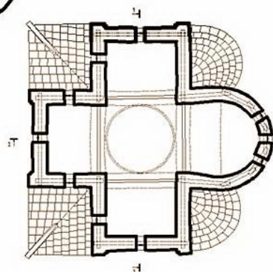
ПЛАН 2 ЯРУСА
