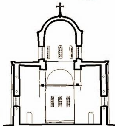
РАЗРЕЗ 1-1
