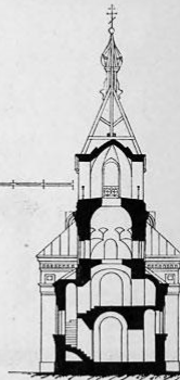
Поперечный разрез колокольни.
