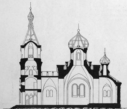
Продольный разрезъ.
