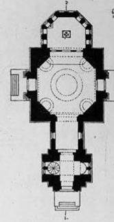
План.
