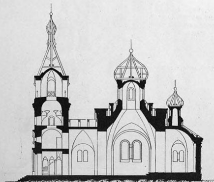
Продольный разрез.
