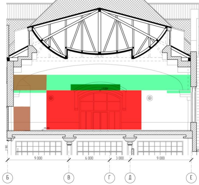
Разрез поперечный по залу
