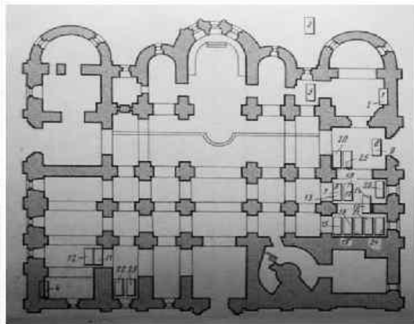
Собор Святой Софии в Новгороде. План (современное состояние)
