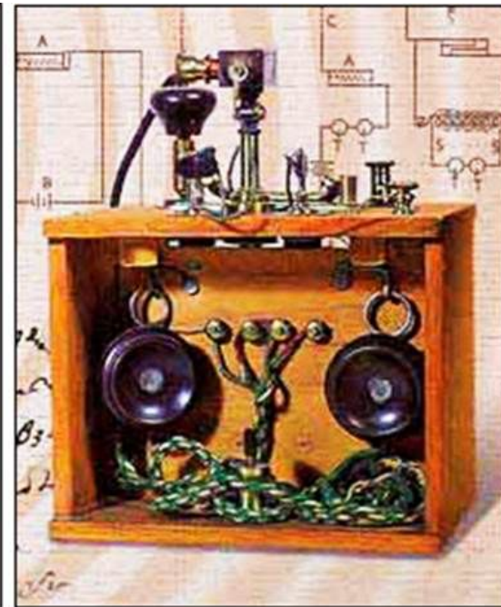
Телефонный приемник системы Попова-Дюкрете 1900
