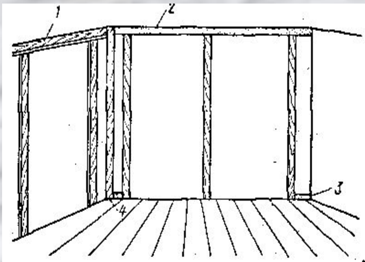
Рис. 50. Устройство лузгов по ранее выполненным маякам:
