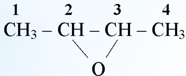
2,3 эпоксидан
