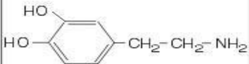
Dopamin
