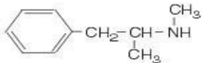
Metamfetamin
