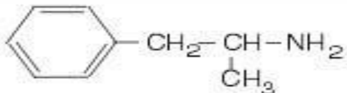
Amfetamin
