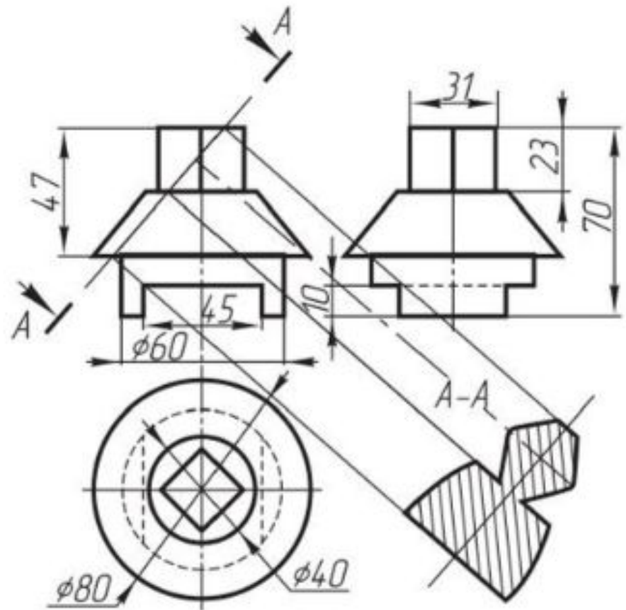
Рисунок 8.5 3D-модель (а) и чертеж с наклонным сечением (б)
