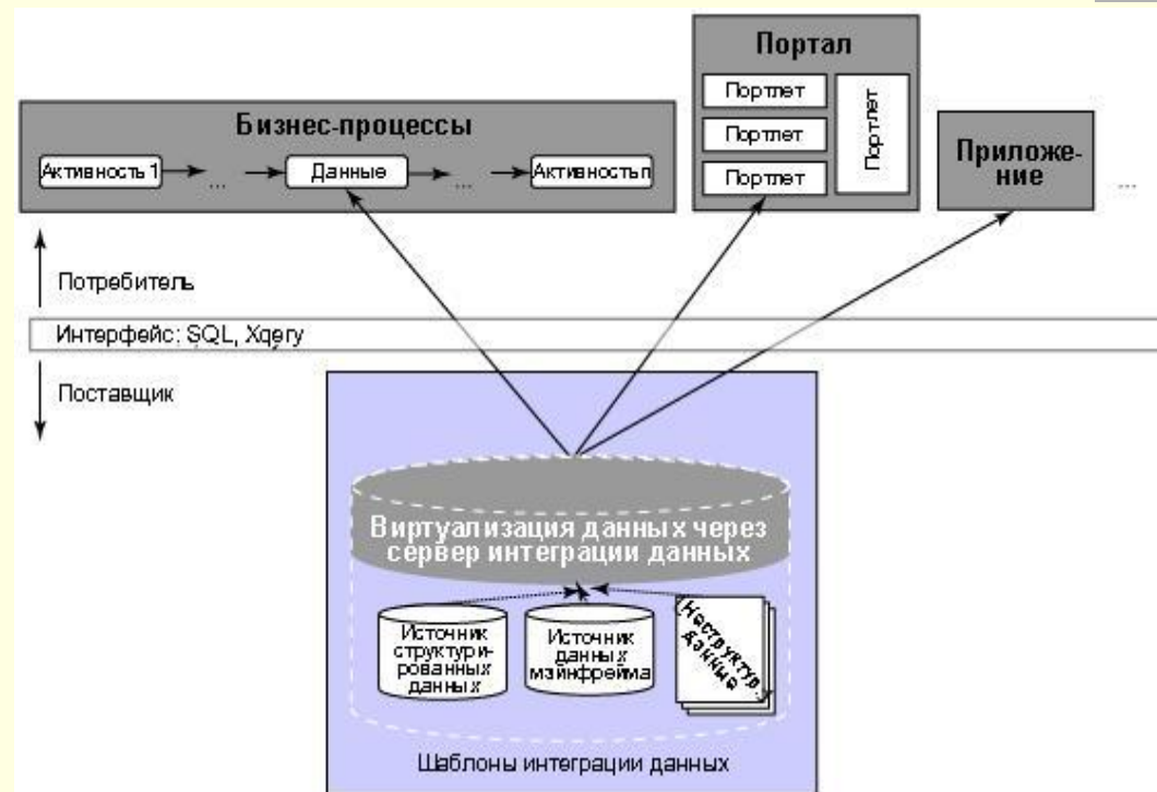
Рисунок 1 - Традиционная схема интеграции данных
