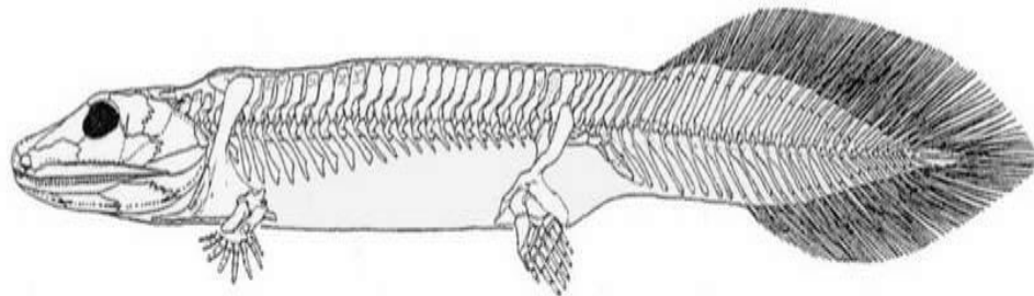
Acanthostegia
