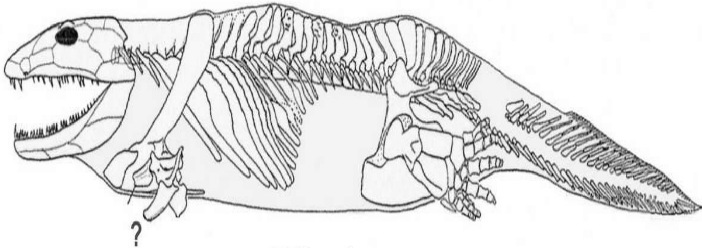
Ichthyostegia
