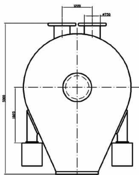
Вид В
