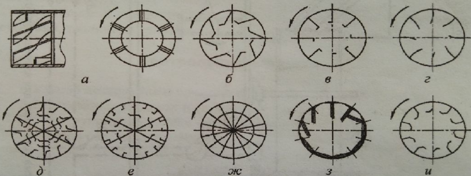
Рис. 13. Схема типов внутренних насадок барабанных сушилок
