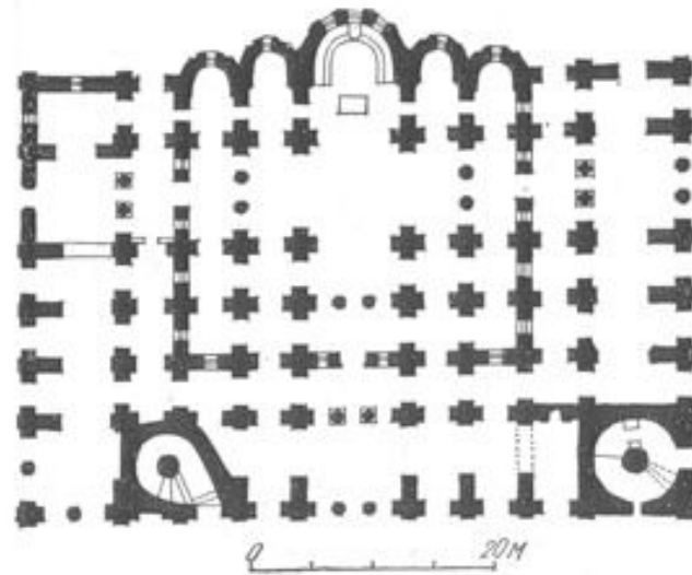
Софийский собор. План. Реконструкция Асеева Ю.С., Кресального Н.И., Волкова В.П.
