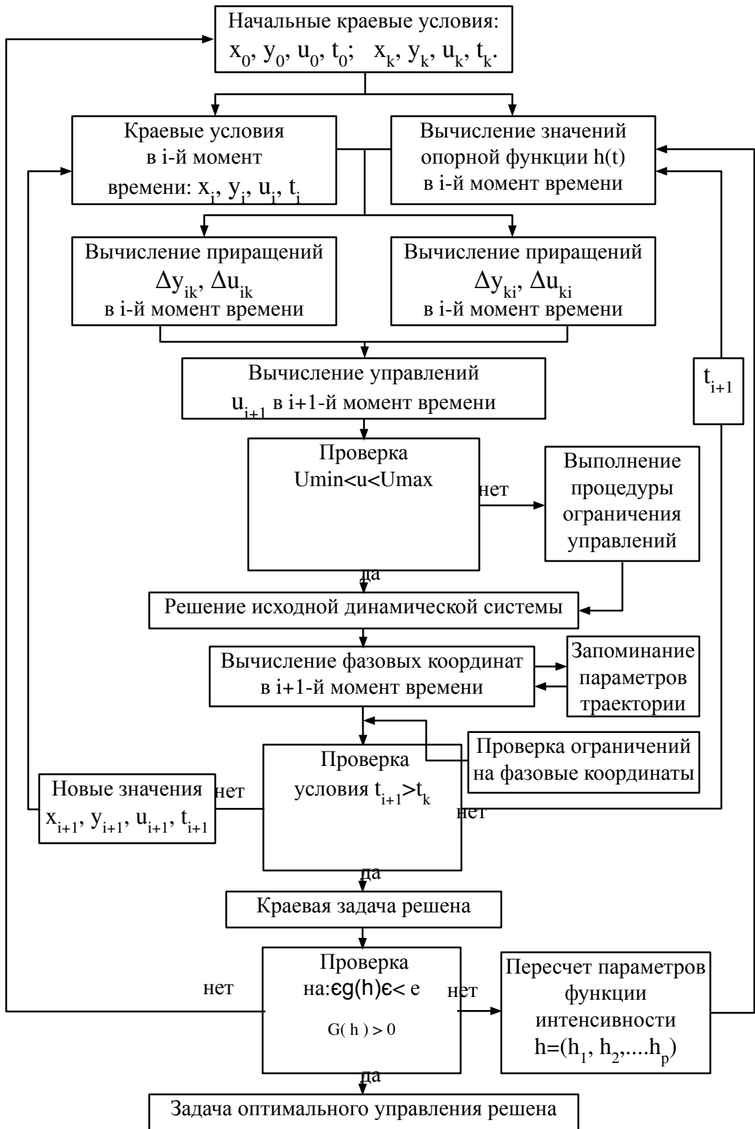
Рис.6.14. Схема алгоритма применения метода прямой оптимизации.
