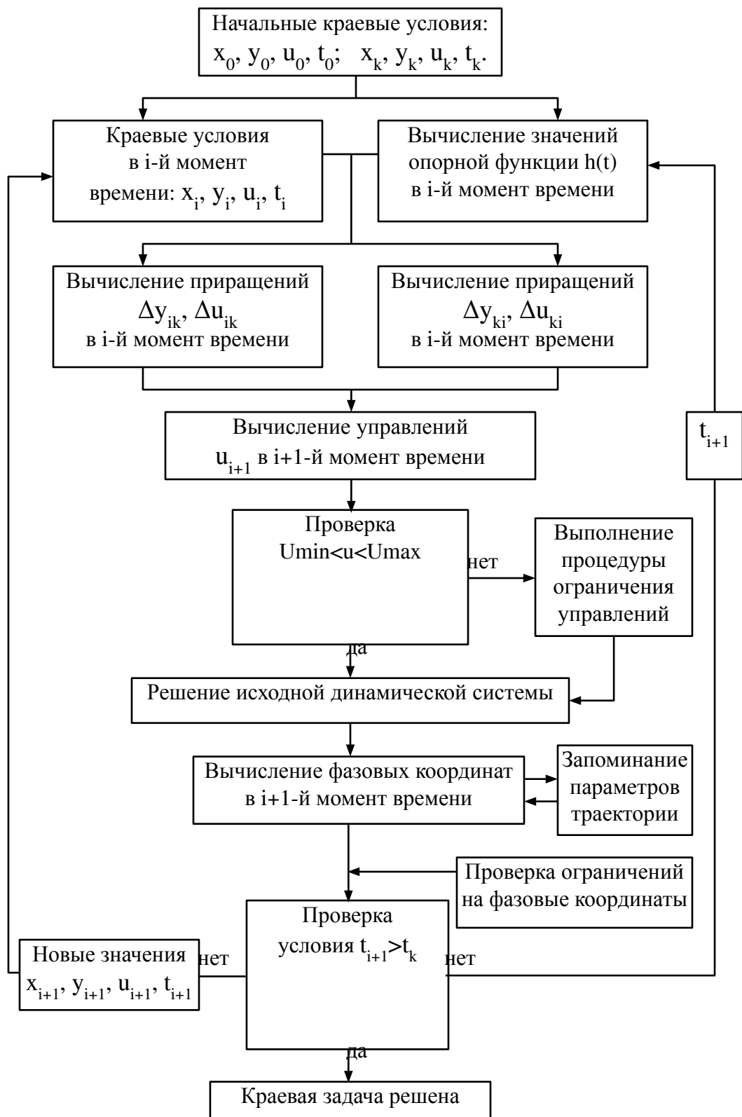
Рис.6.14. Алгоритм применения разностной схемы метода к решению краевых задач.
