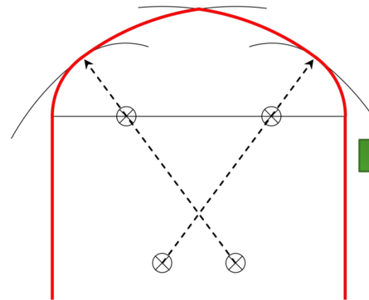
Четырёхцентровая арка (арка Тюдоров)
