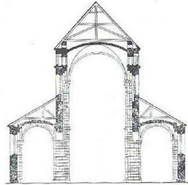
Поперечный разрез романского базиликального храма (собор в Шпейере, XI-XII в.)
