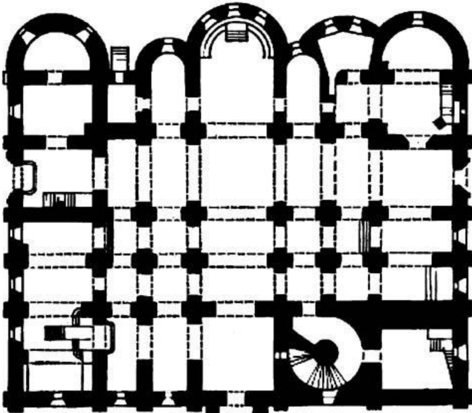
План собора Св. Софии в Новгороде. 1045-1050.
