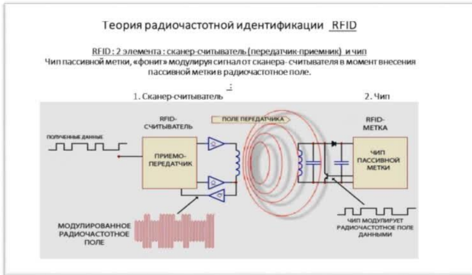
Рисунок 6 Теория радиочастотной идентификации
