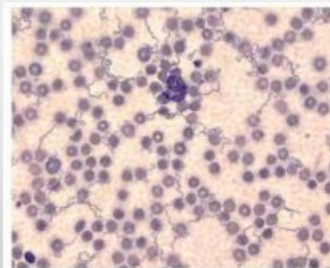
Borrelia recurrentis Мазок крови во время приступа
