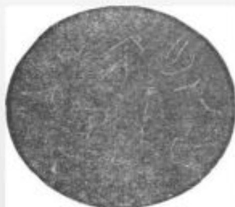
Leptospira. Тушевой мазок по Бурри
