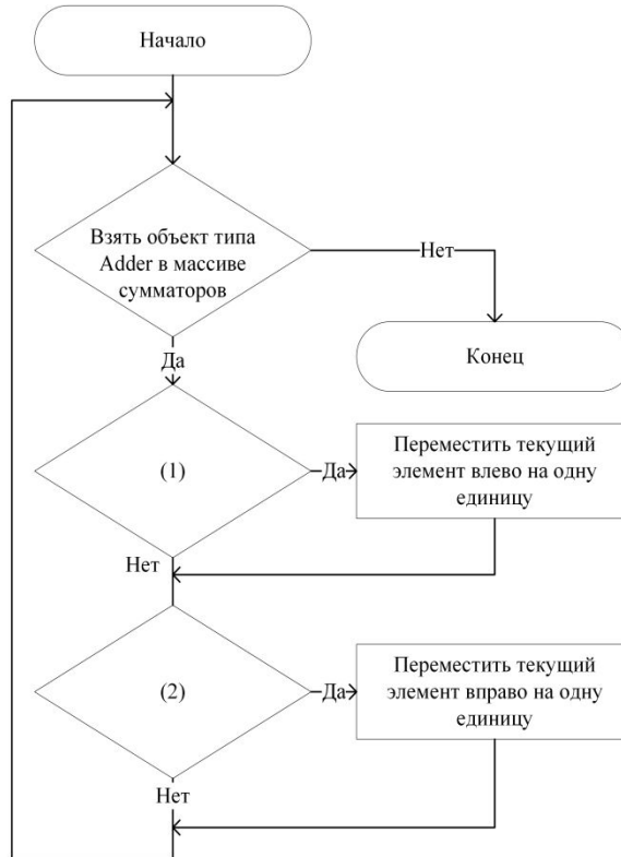
Перемещение сумматора
