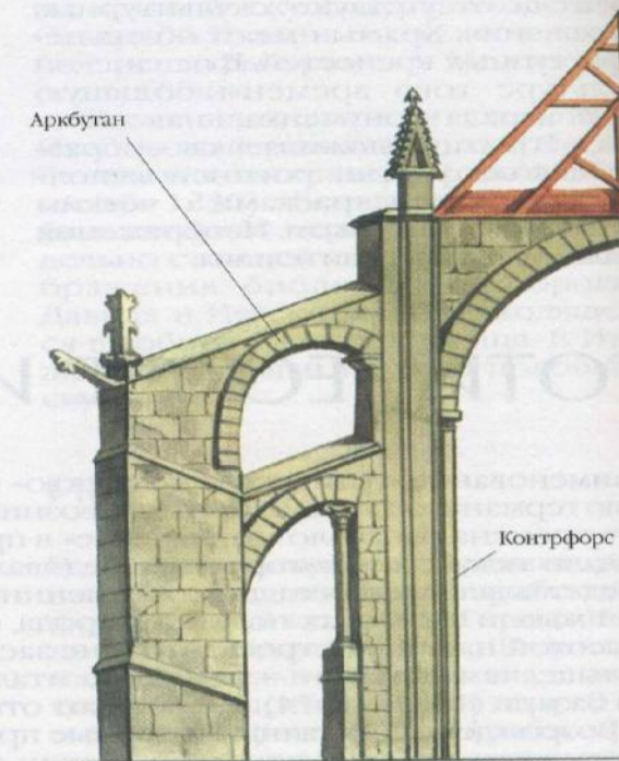
Система аркбутанов и контрфорсов.
