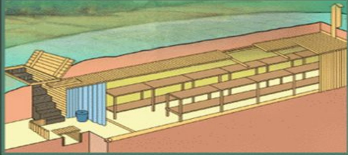
Противорадиационное укрытие
