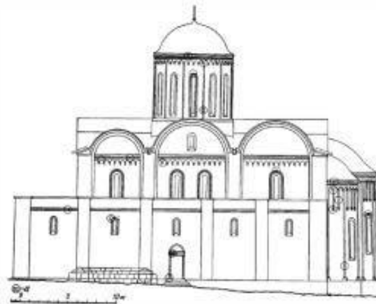
Реконструкция южного фасада Успенского собора в Галиче А.А.Тица.
