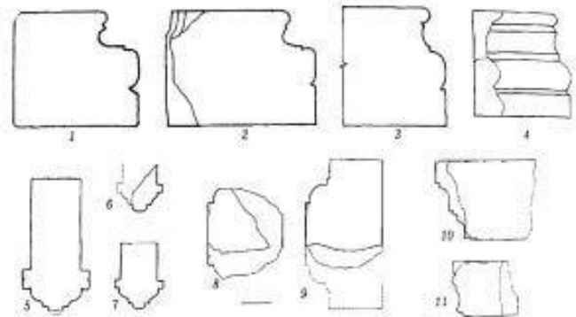
1 - алебастровая база со стены 48; 2 - алебастровая база со стены 17; 3 - известняковая база, сохранившаяся in situ в наземной стене 48; 4 - известняковая база, обнаруженная в Старостинском замке в Галиче; 5-7 - профили нервюр; 8-9 - вертикальные элементы; 10-11 - карнизные профили.
