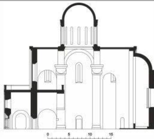
Успенский собор в Галиче. Продольный разрез: Реконструкция. Ardruss.ru.
