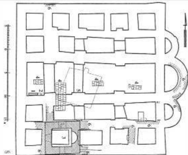
План Успенского кафедрального собора древнего Галича в Крылосе по Я.И.Пастернаку.
