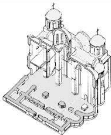
Вариант объемно-пространственной реконструкции Успенского собора на 2-й строительный период - первая треть XIII - начало XVI в. Рис. В. Петрика.
