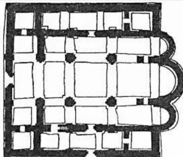
Реконструкция плана Успенского собора в Галиче Ю.В.Лукомского.
