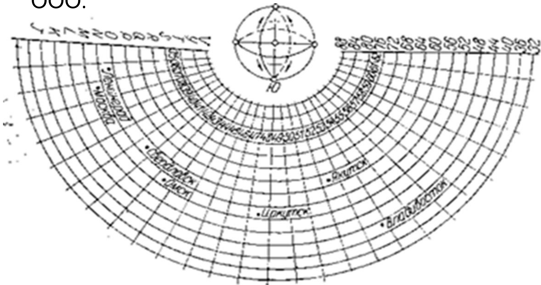
Рис. 51. Международная разграфка листов карт масштаба 1 : 1 000 000.
