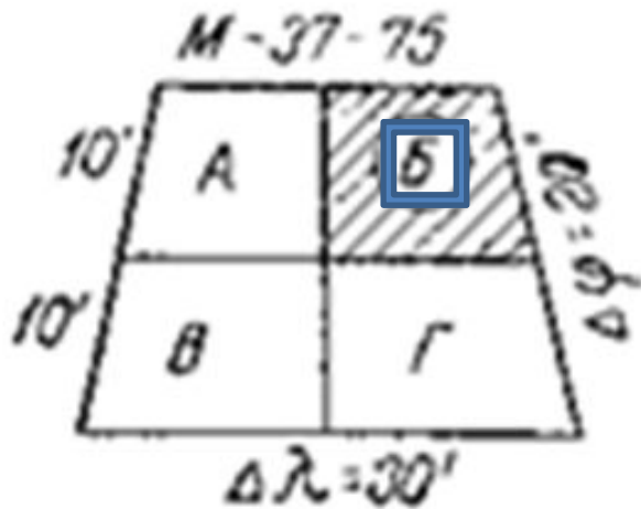
Рис. 54. Разграфка листа карты масштаба 1:100 000 на листы карты масштаба 1:50 000.
