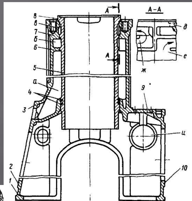
Блок-картер
