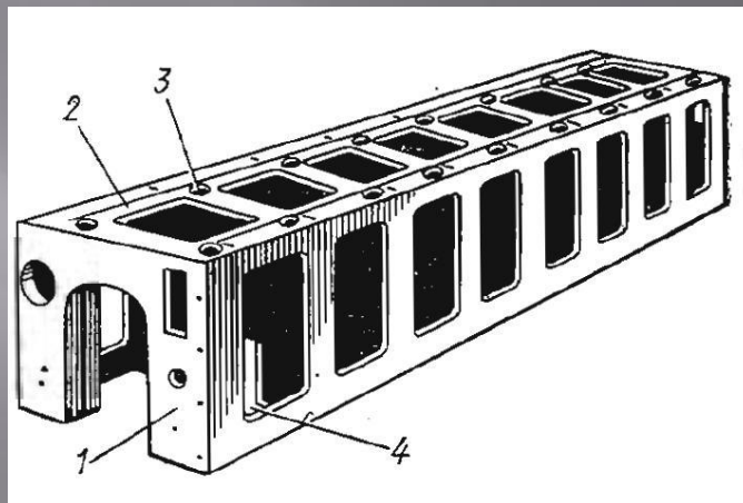
Станина коробчатой формы тронкового дизеля
