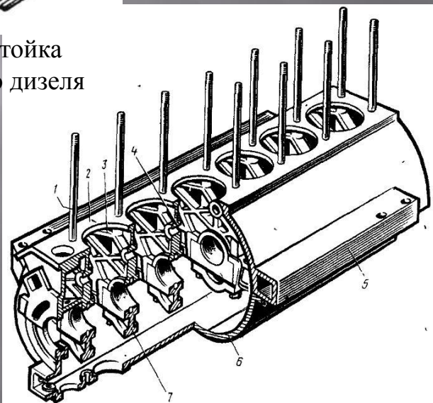
Несущий картер
