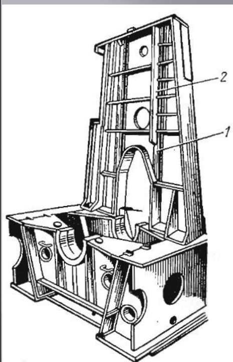
А-образная стойка крейцкопфного дизеля
