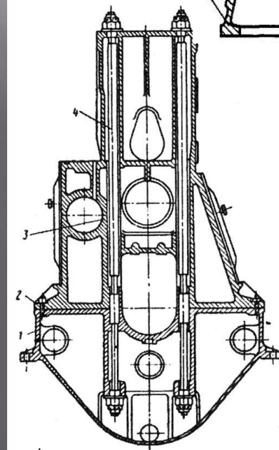
Анкерное крепление деталей остова дизеля
