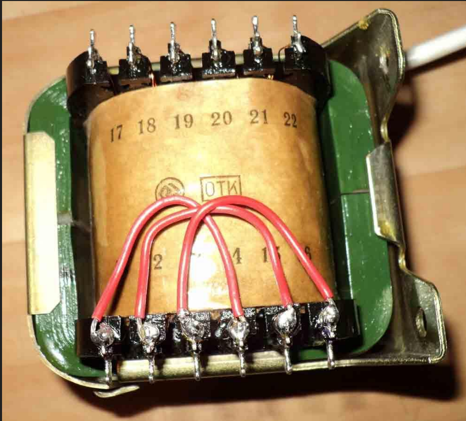
Припаивание проводов к выводам трансформаторов
