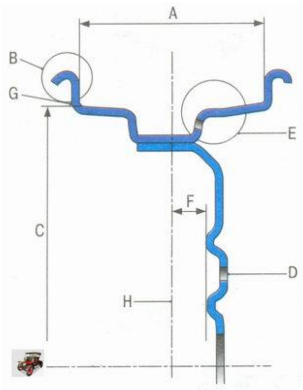
Параметры колесных дисков Лада Гранта
