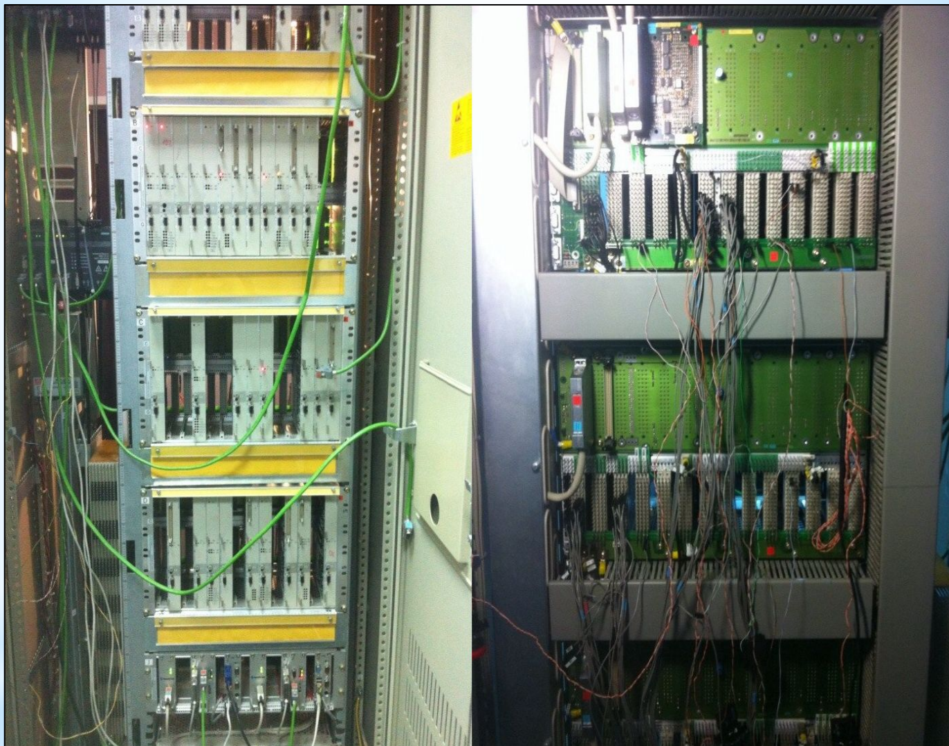
* Внешний вид БШС ТПТС-51
