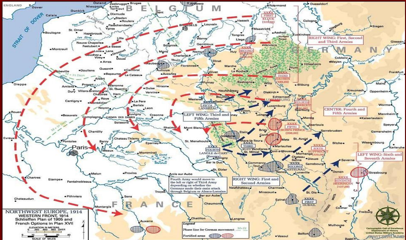
Диаграмма, показывающая общую идею плана Шлиффена 1905 года (отличного от применяемого в 1914 году).
