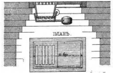
ФИГ. 7 СТОЧНЫЙ ДВОРОВЫЙ КОЛОДЕЦЪ - РАЗРѢЗЪ
