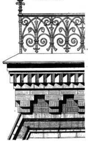
ФИГ. 10 ДЕТАЛЬ БАЛКОННОЙ РЕШЕТКИ И КАРНИЗА
