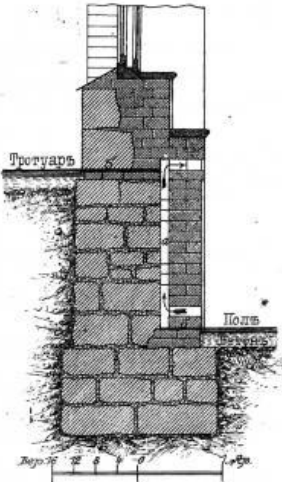
ФИГ. 6 СТЫННАЯ ФОРТОЧКА 1/4 Науры
