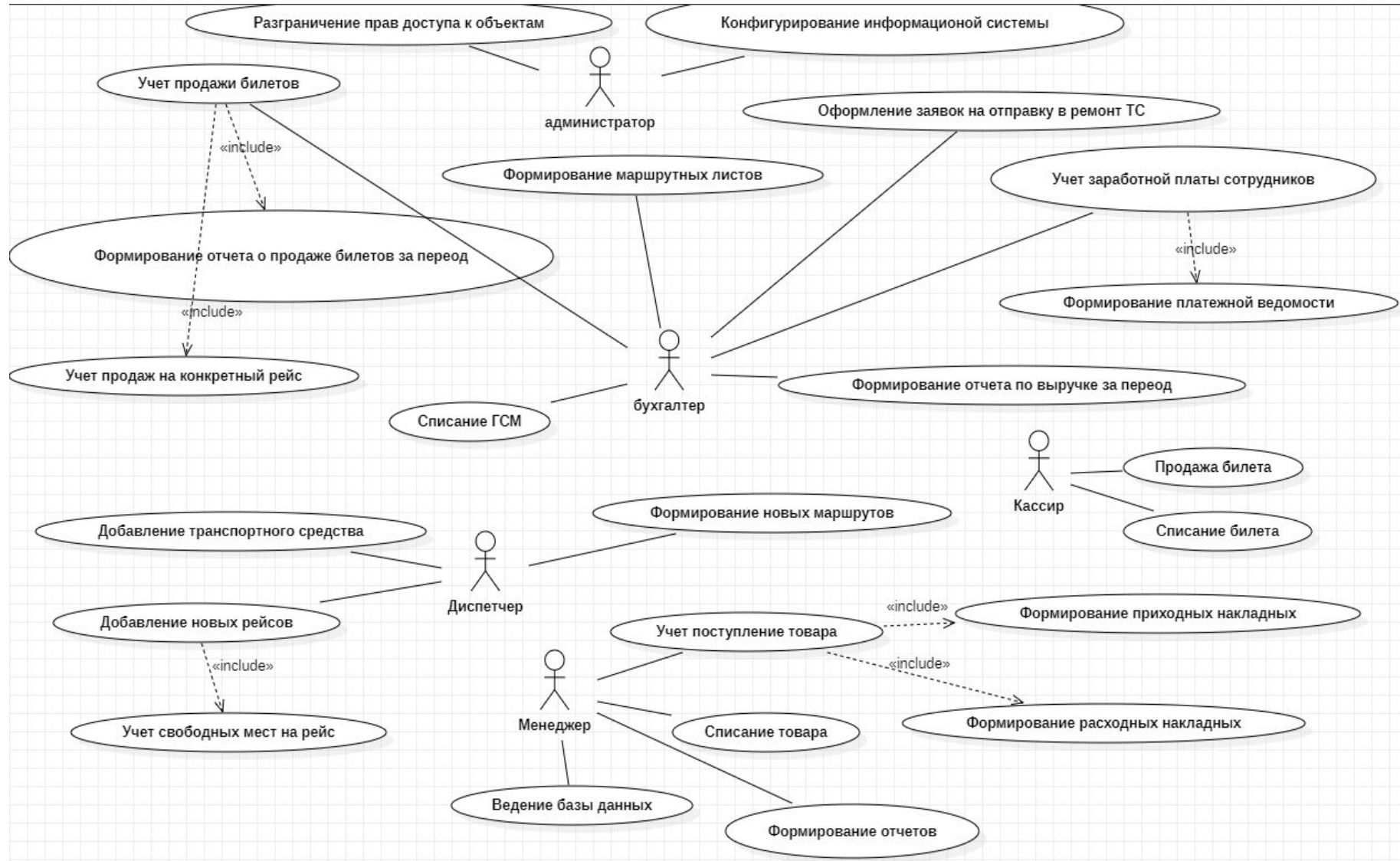
Рисунок 2 – Диаграмма вариантов использования
