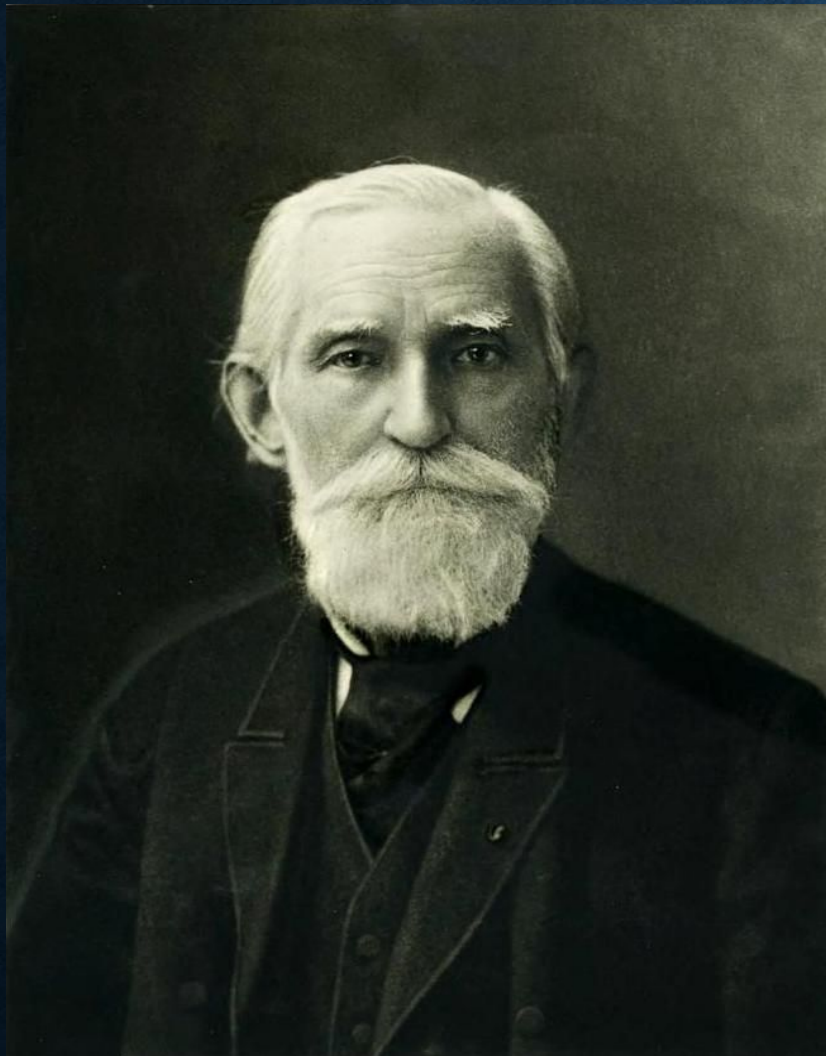
Чебыше В
