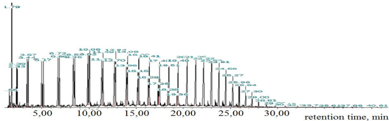
Хроматограмма парафина после облучения электронами
