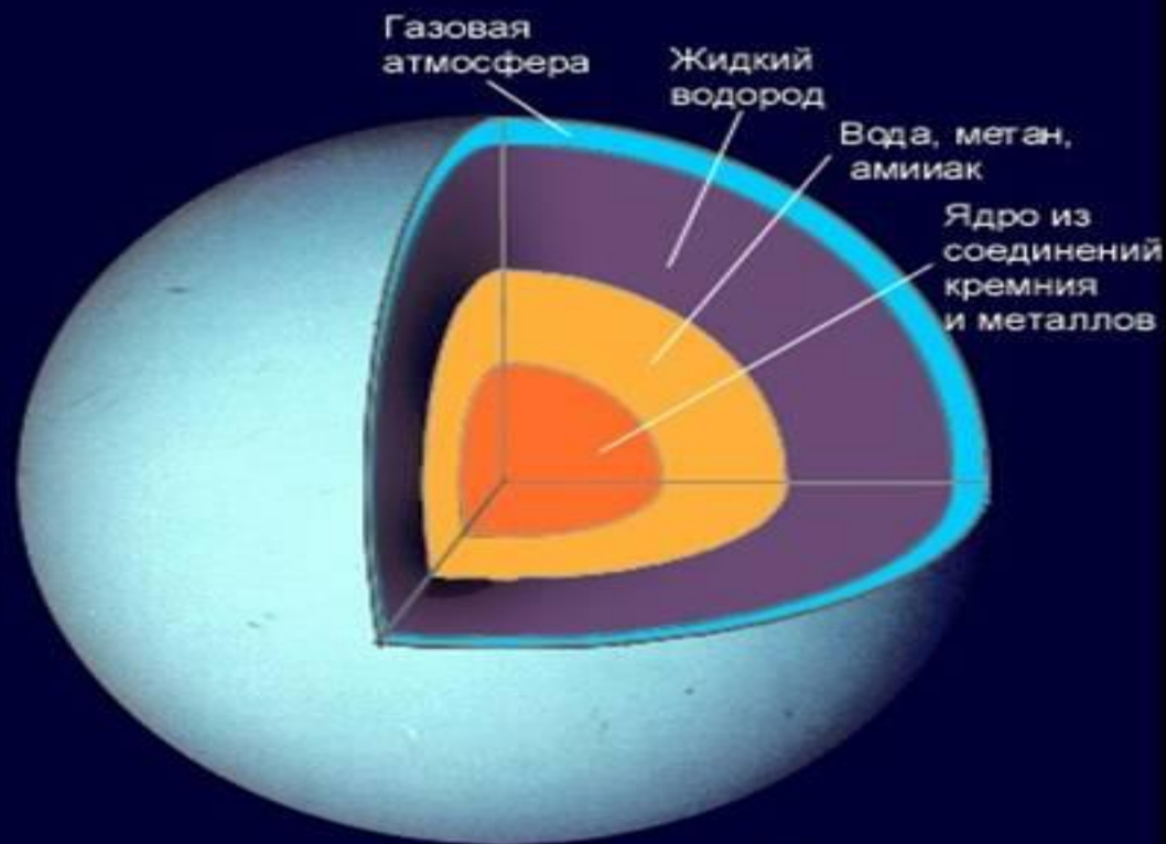
Внутреннее строение Урана
