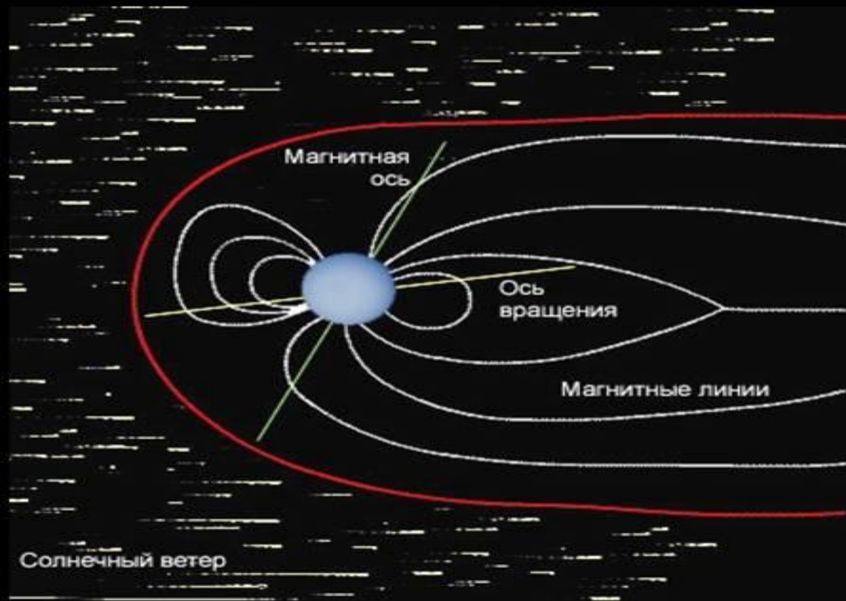
Магнитосфера Урана
