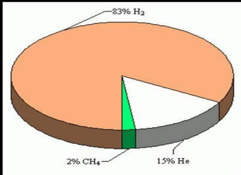
Химический состав атмосферы Урана
