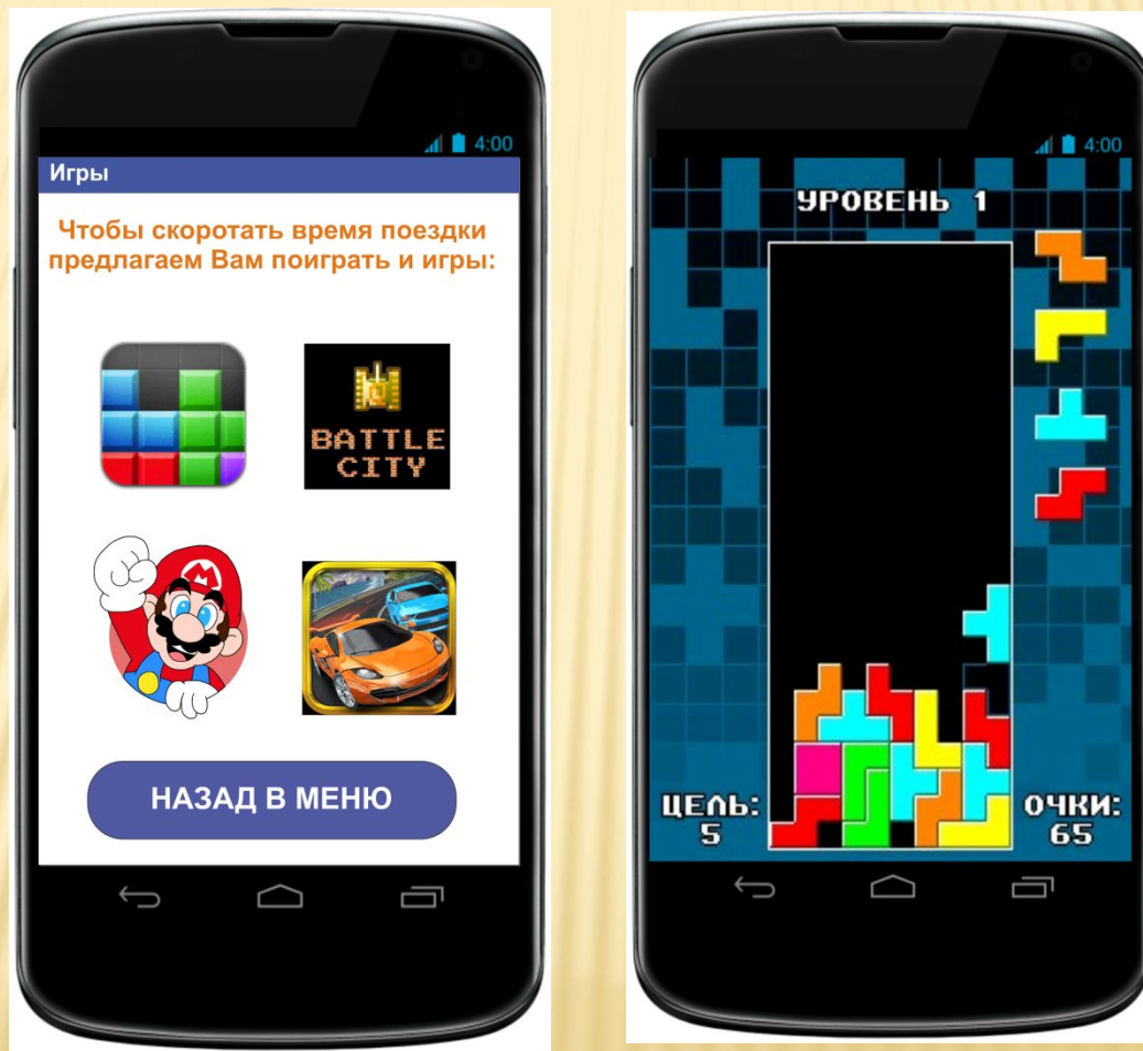
Рис. 7 Мини-игры
