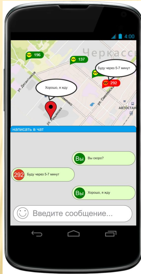
Рис. 6 Оценка водителя
