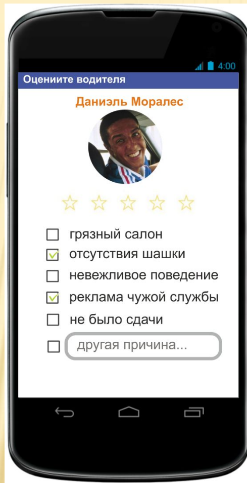
Рис. 8 Оценка водителя
