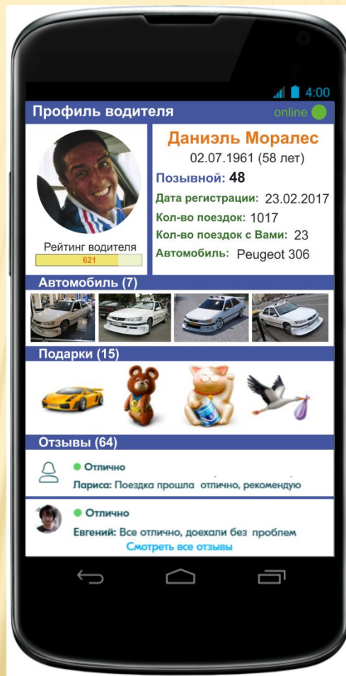
Рис. 5 Профиль водителя
