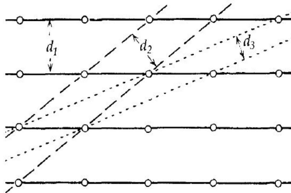
Рис. 10.4. Схема, иллюстрирующая различные межплоскостные расстояния ( d ) в структуре кристалла
