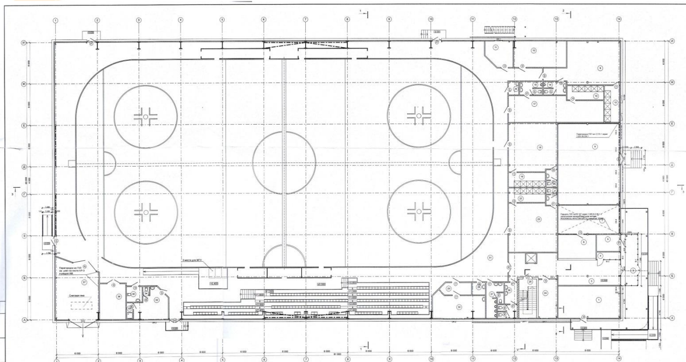
Экспликация помещений 1-го этажа
