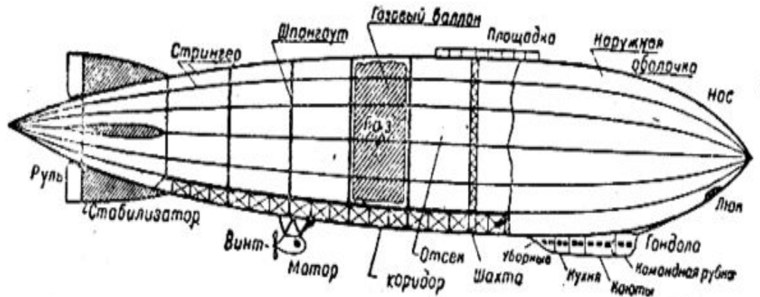
Рис. 11. Схема дирижабля жесткой системы (типа цеппелин).
