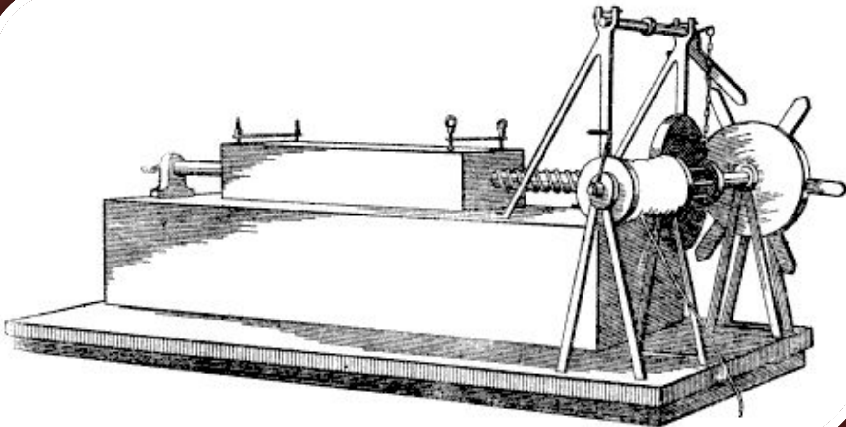
Станок для насечки напильников
