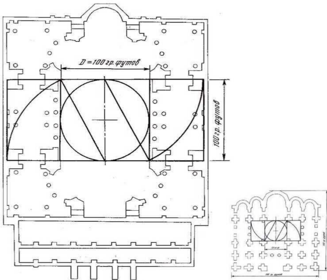
Планы Софии Константинопольской и Софии Киевской (по К.Н. Афанасьеву)
